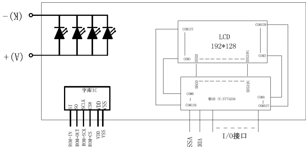
图 2：JLX192128G-971-PL 电路框图
