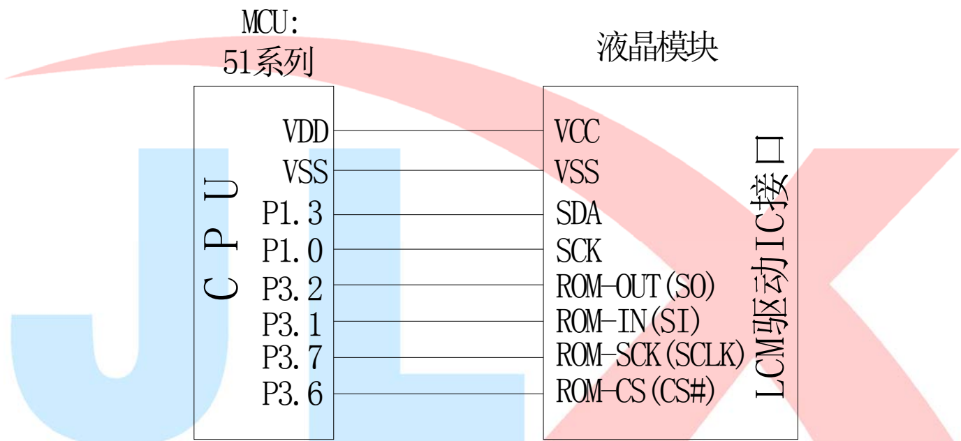
图 3：IIC 接口图
