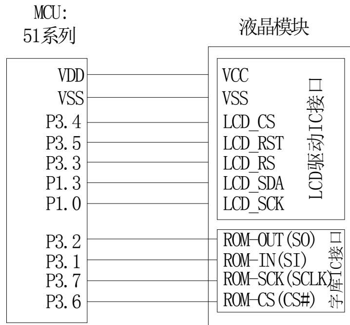
图 2：串行接口图
