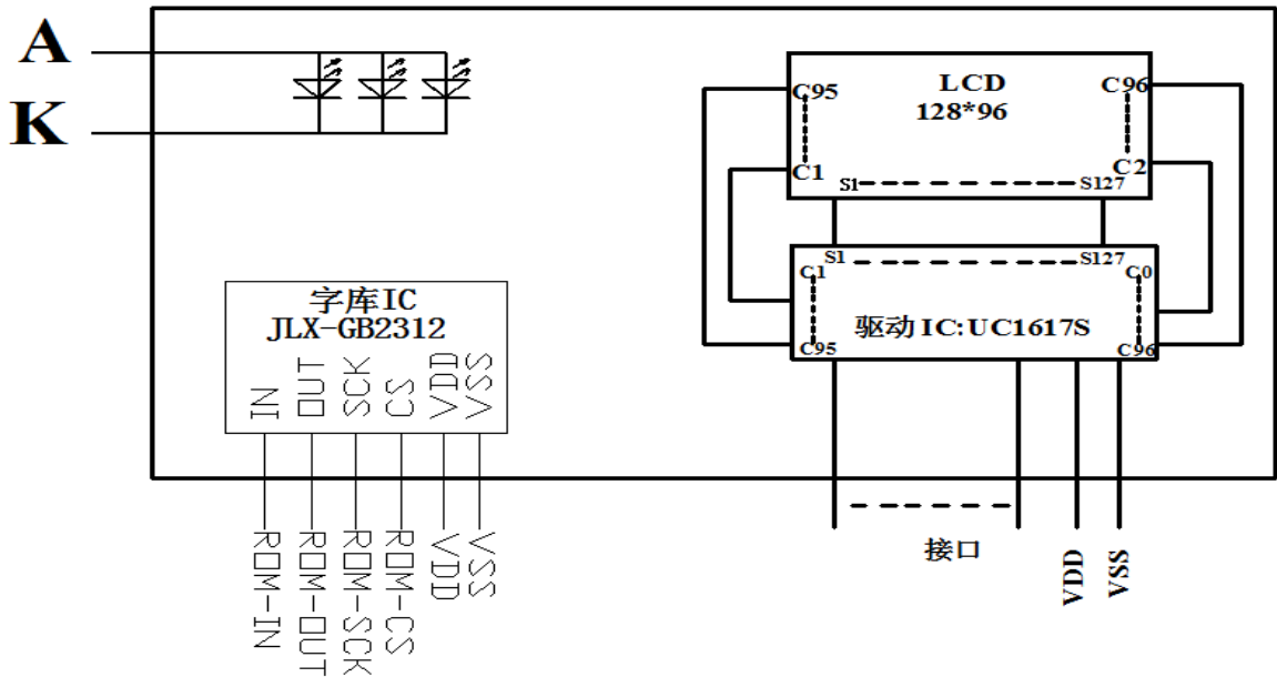
图 2: 电路框图
